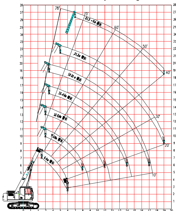
Grue SWTC10 - Hauteur et rayon de levage
